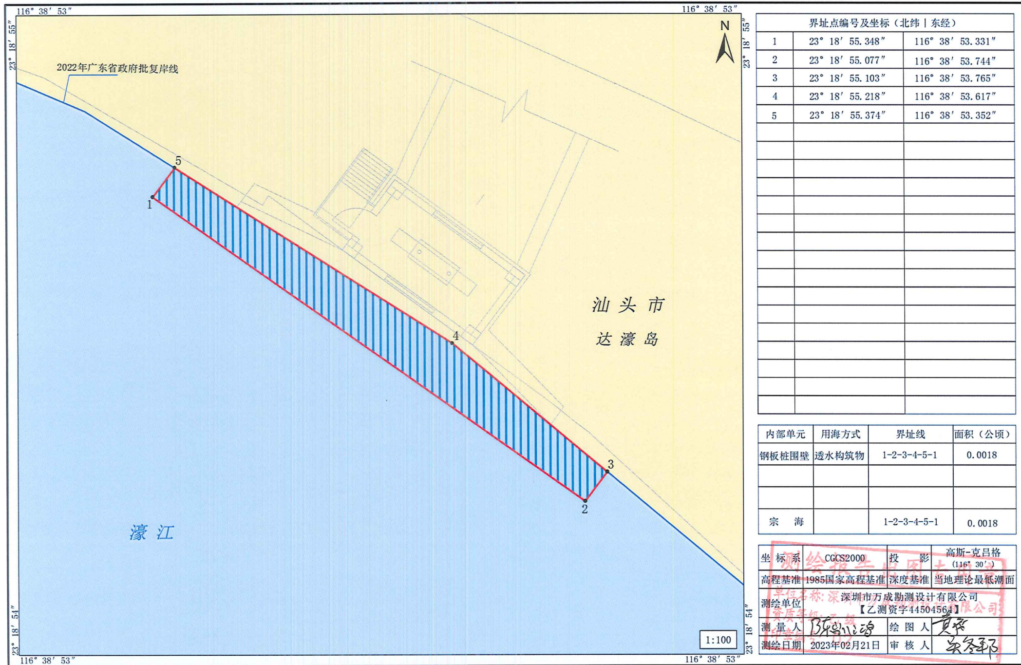
濠江北路（磊口大桥-河浦花桥）道路建设工程、濠江北路（河浦花桥-达南路）道路建设工程项目临时用海(磊口段)宗海界址图
