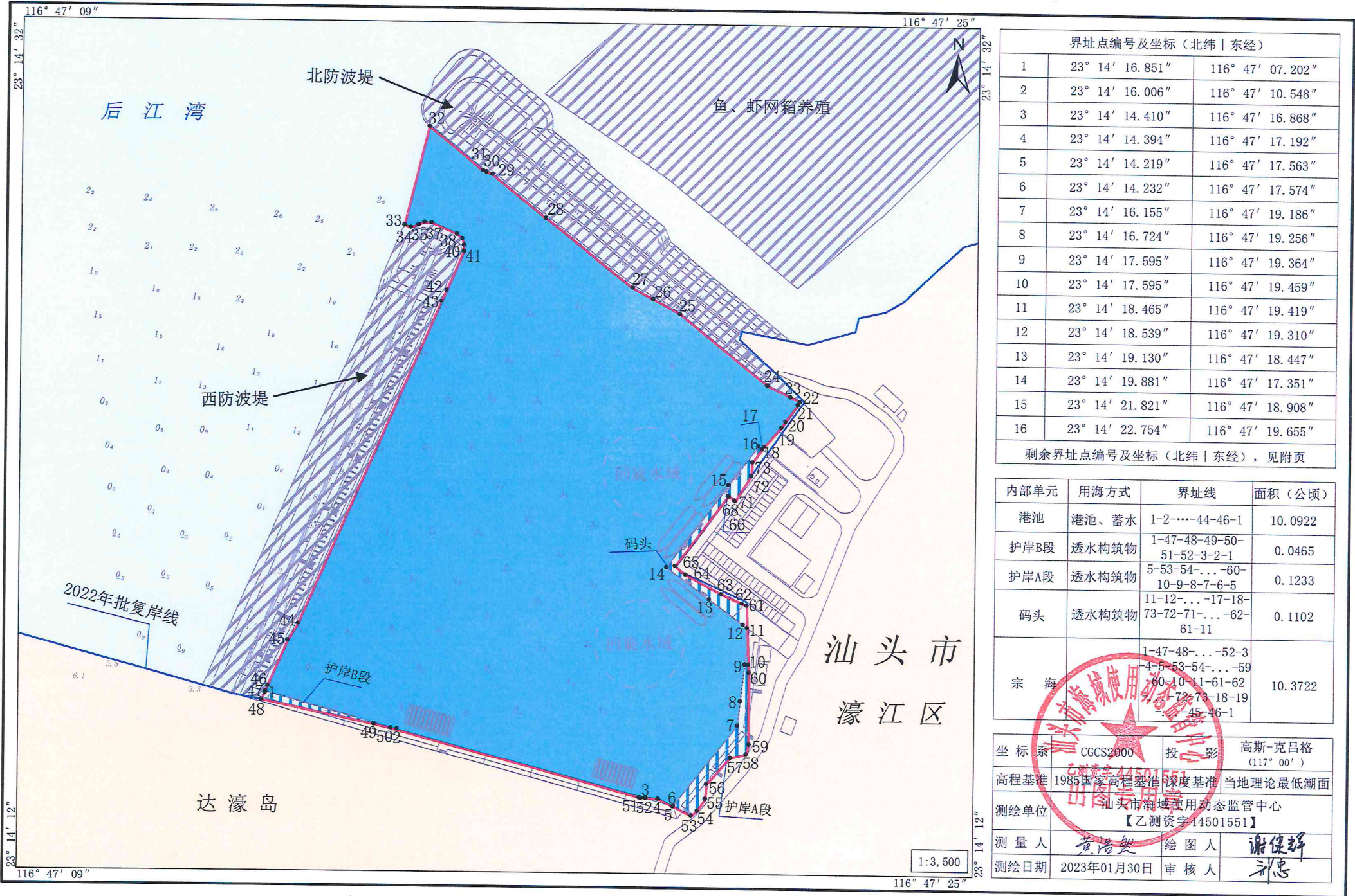
广澳后江乡镇渔港建设项目（港池、护岸、码头）宗海界址图
